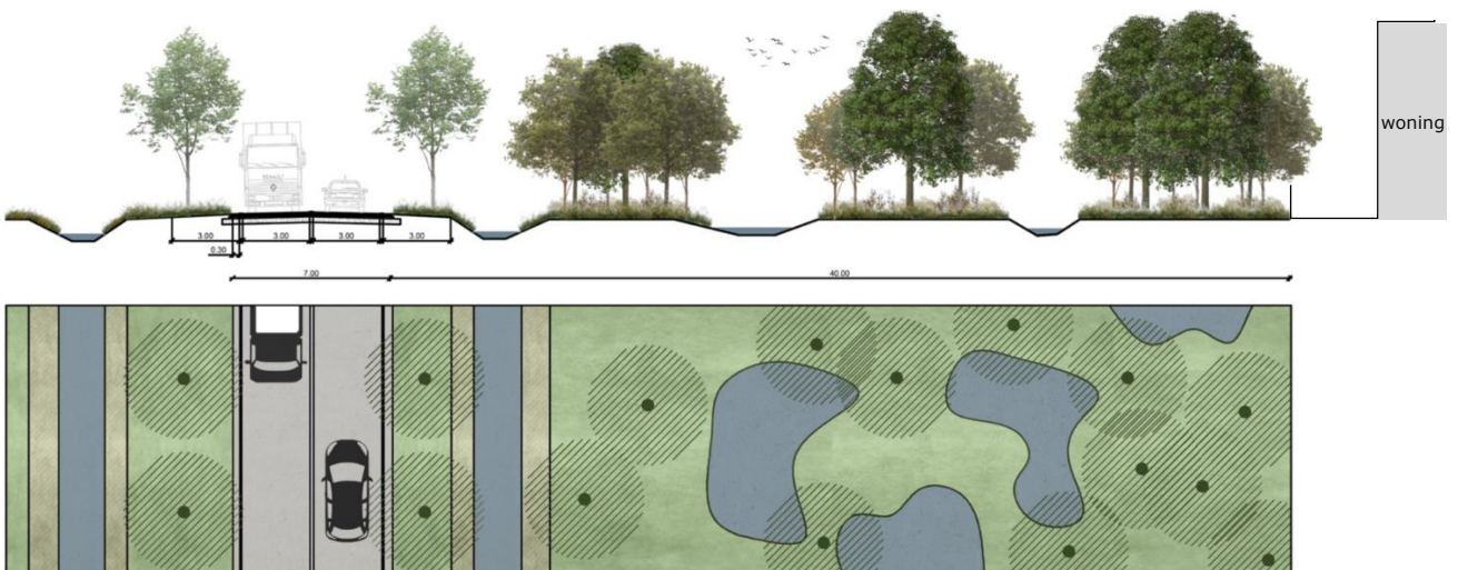
Figuur 44: Schematische doorsnede van de groenbuffer tussen de nieuwe weg en de bestaande woningen aan de Witbol-, Lupinen- en Spurriestraat, Koppeleershoeven, Gagel- en Heistraat.
